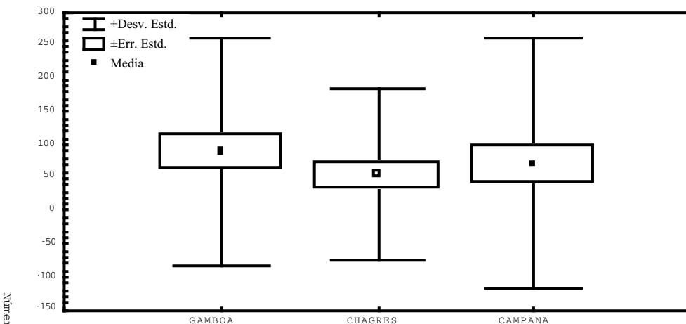
Figura 2. El diagrama de caja muestra el valor promedio (media), la desviación estándar (desv. estd.), el error estándar (err. estd.) de las muestras obtenidas en los sitios seleccionados.
